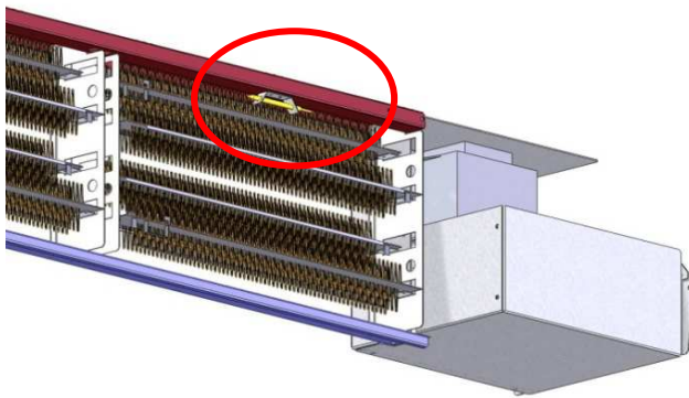
Kuva termostaattin sijainnista – Ditrionic-ohjain
