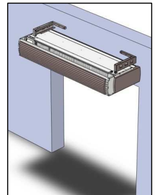
Asennus vaakasuuntaan – seinälle
