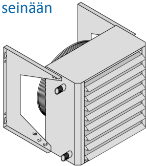
Asennus seinään
