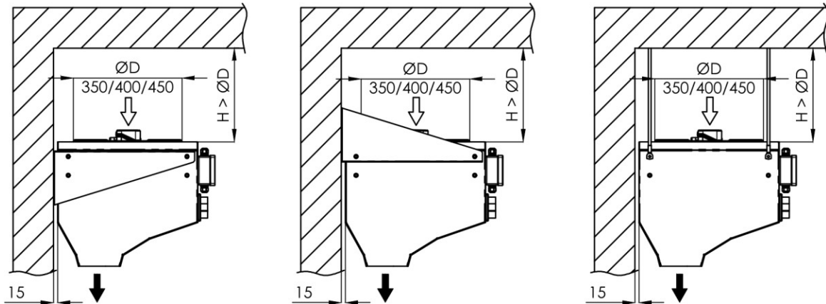
Asennusetäisyys yksikkötyypeittäin
