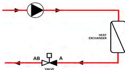
Liitäntä, kaksitieventtiili TV, ETVQ
